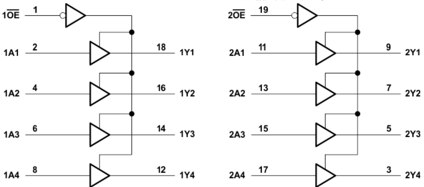
図 3-1. 概略回路図
