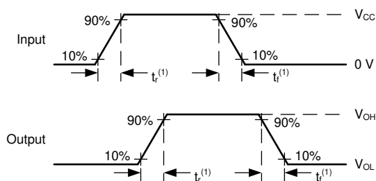
図 6-3. 電圧波形、入力と出力の遷移時間
