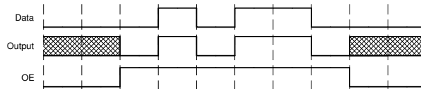
図 8-2. アプリケーションのタイミング図
