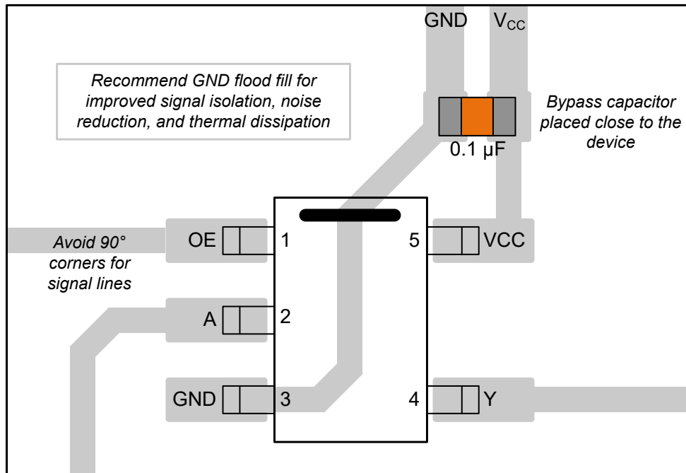
図 8-3. SN74LV1T126-Q1 のレイアウト例
