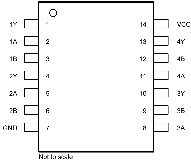
図 4-1. PW パッケージ、14 ピン TSSOP (上面図)
