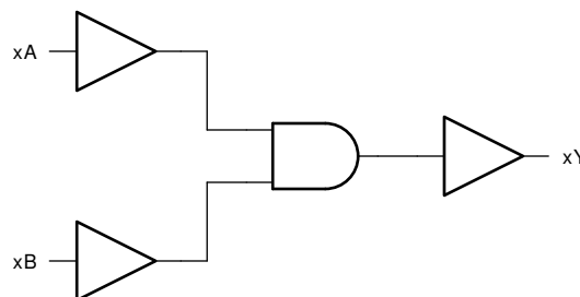
概略論理図 (正論理)
