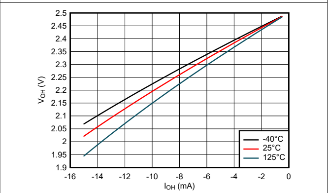
図 5-4. High 状態における出力電圧と電流との関係、2.5V 電源
