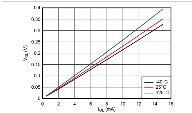
図 5-5. Low 状態における出力電圧と電流との関係、2.5V 電源
