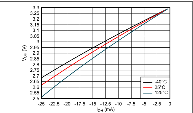
図 5-2. High 状態における出力電圧と電流との関係、3.3V 電源
