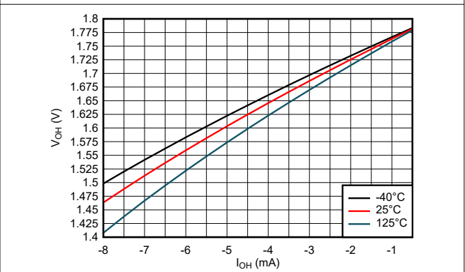
図 5-6. High 状態における出力電圧と電流との関係、1.8V 電源
