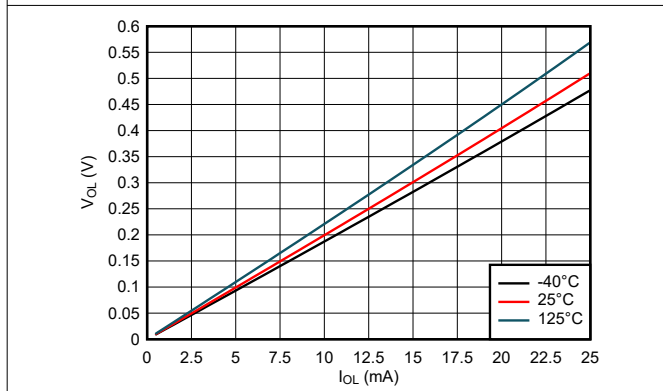
図 5-3. Low 状態における出力電圧と電流との関係、3.3V 電源
