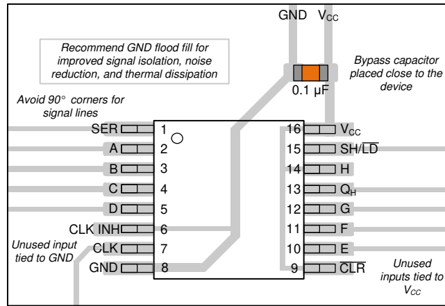
図 8-3. SN74LVC166A のレイアウト例
