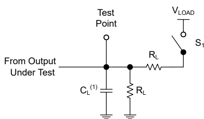
図 6-1. オープン ドレイン出力の負荷回路
