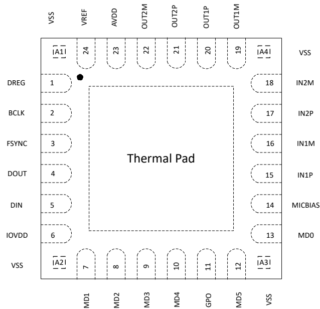
図 5-1. TAC5142 Pinout
