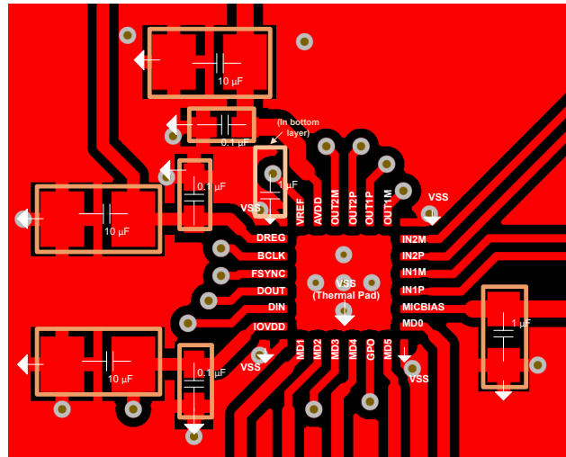
8-7. Example Layout
