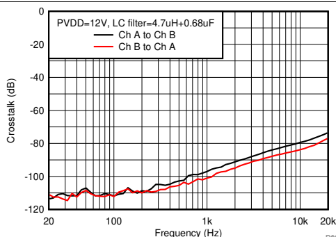
图 26. Crosstalk
