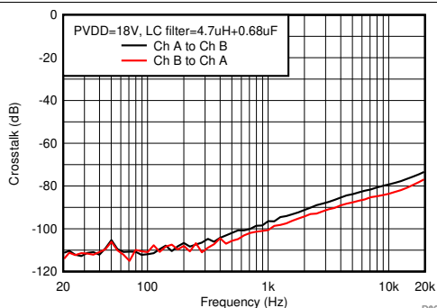
图 28. Crosstalk
