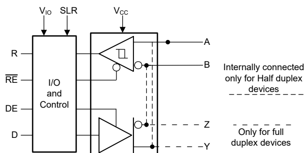
概略回路図
