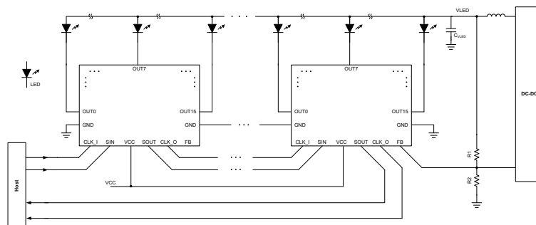
簡略回路図
