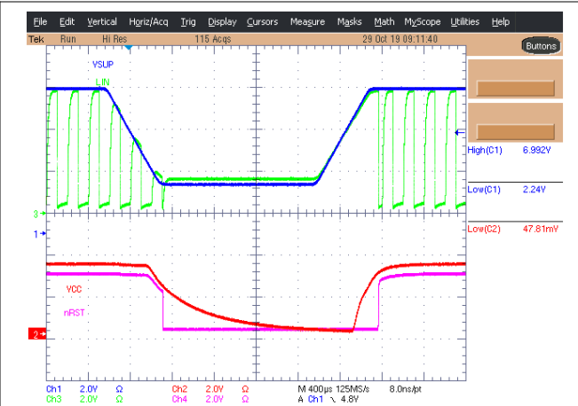
10-9. TLIN10283S-Q1 Brownout
