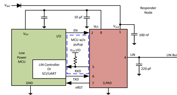
概略回路図、レスポнда・ノード(2)
