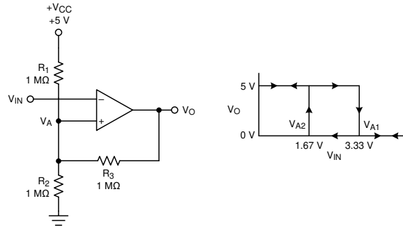
图 8-3. TLV185x 在具有迟滞的倒相配置中
