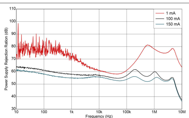
図 7-3. PSRR
