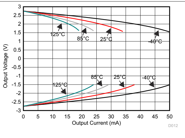
図 7-12. 出力電圧と出力電流との関係 (クロウ)
