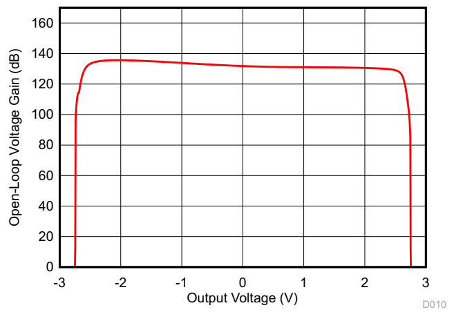
図 7-10. 開ループのゲインと出力電圧との関係
