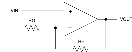
図 7-3. 回路図
