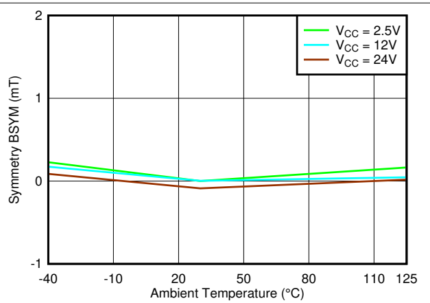
图 7-62. B_{SYM}(y) vs. Temperature
