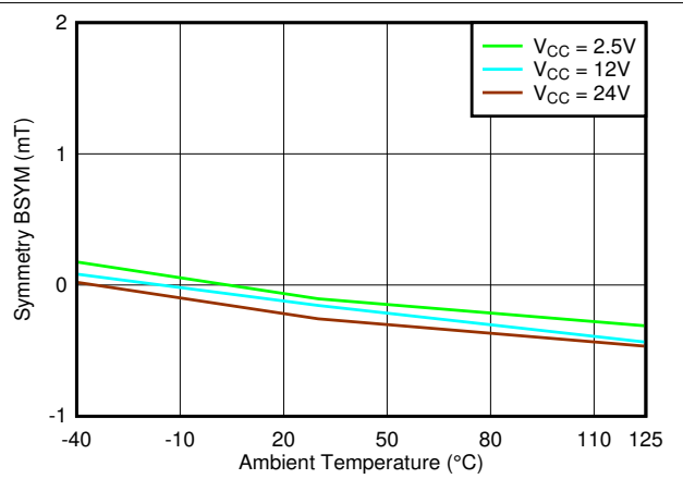
图 7-60. B_{SYM}(x) vs. Temperature
