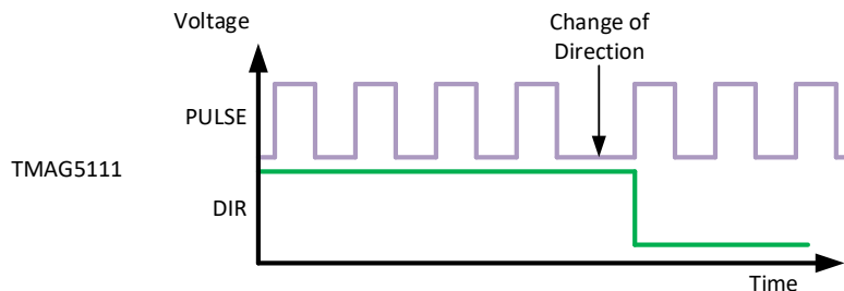
图 9-3. TMAG5111 Output Response
