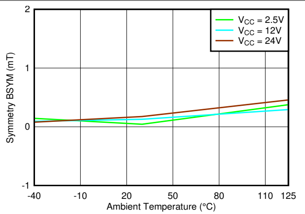
图 7-58. B_{SYM}(z) vs. Temperature
