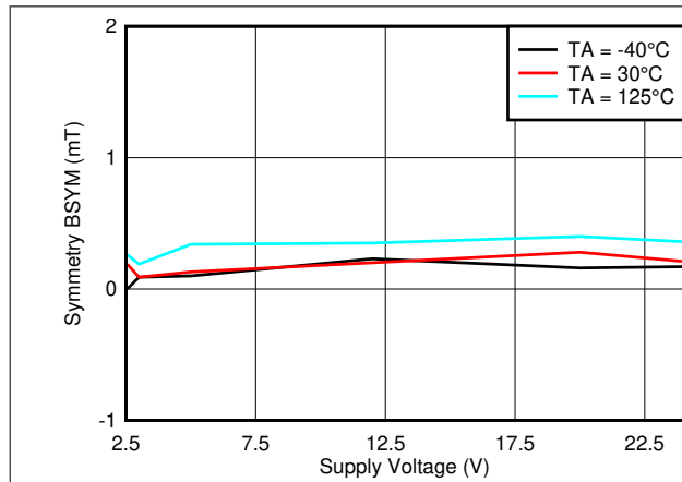
图 7-19. B_{SYM(Z)} vs. V_{CC}
