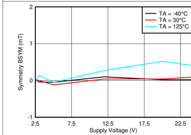
图 7-21. B_{SYM(X)} vs. V_{CC}
