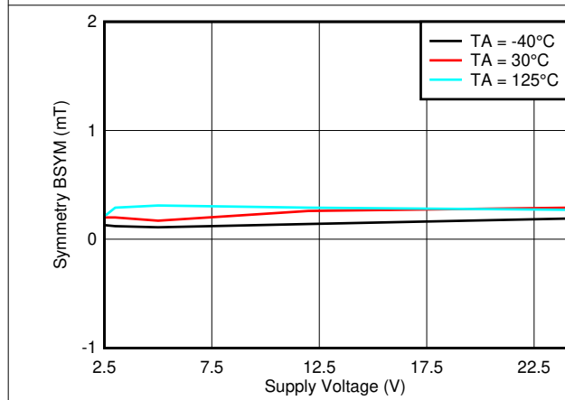
图 7-23. B_{SYM(Y)} vs. V_{CC}
