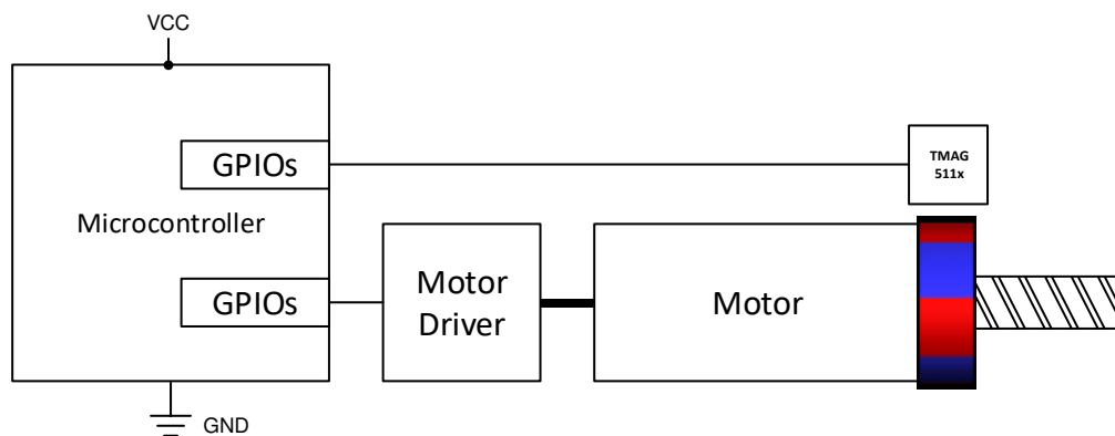
図 9-1. Incremental Encoding
