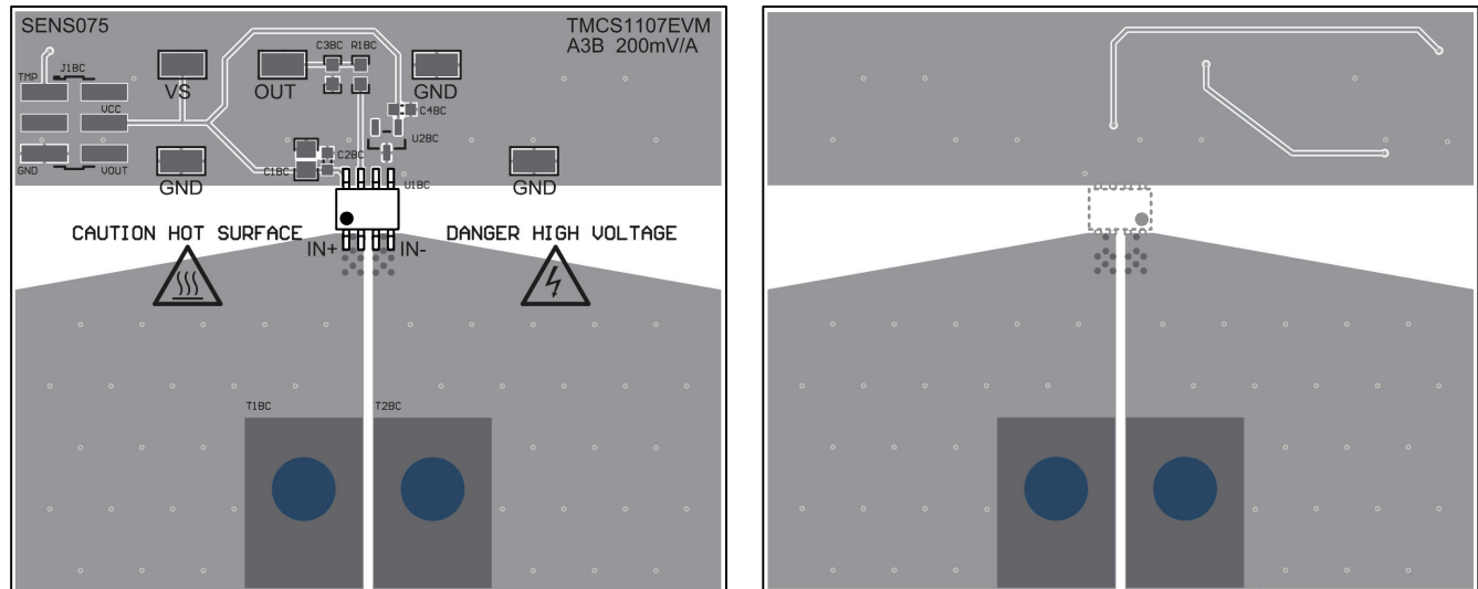
図 12-3. 基板の上表面 (左) と底面 (右) プレーンの推奨レイアウト
