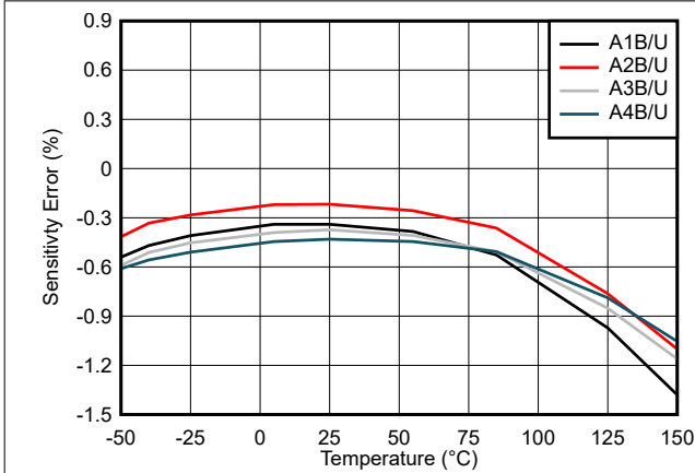
図 7-1. TMCS1107-Q1 感度誤差と温度との関係
