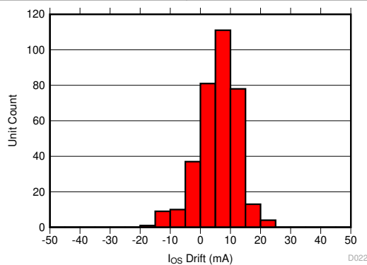
図 9-3. AEC-Q100 高温動作寿命ストレス・テスト後の入力換算オフセット・ドリフト
