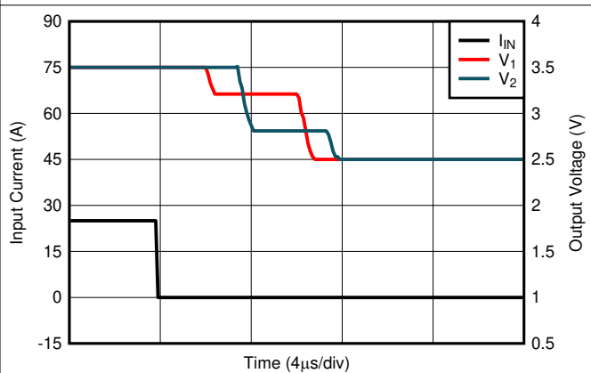
図 7-10. 電圧出カステップ、立ち下がり
