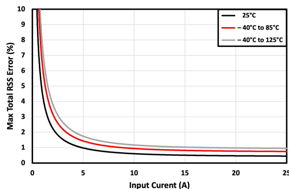
图 9-1. RSS Error vs Input Current
