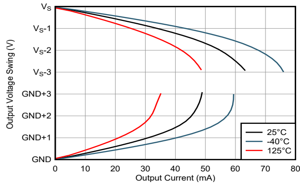
图 6-21. Output Swing vs Output Current
