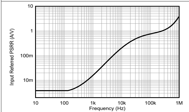
図 6-15. PSRR vs Frequency
