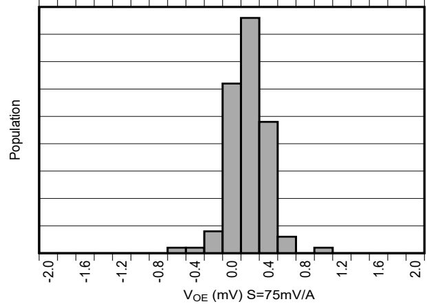
図 6-8. Offset Error Production Distribution
