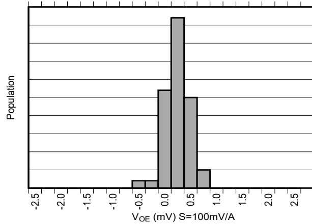
図 6-9. Offset Error Production Distribution
