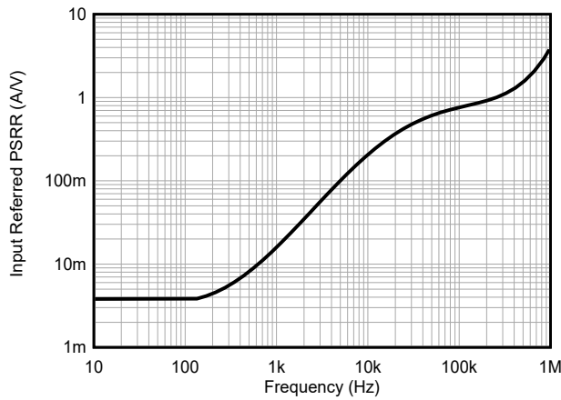
図 6-9. PSRR vs Frequency
