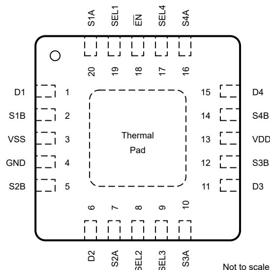
図 5-2. TMUX6234 RRQ Package, 20-Pin WQFN (Top View)
