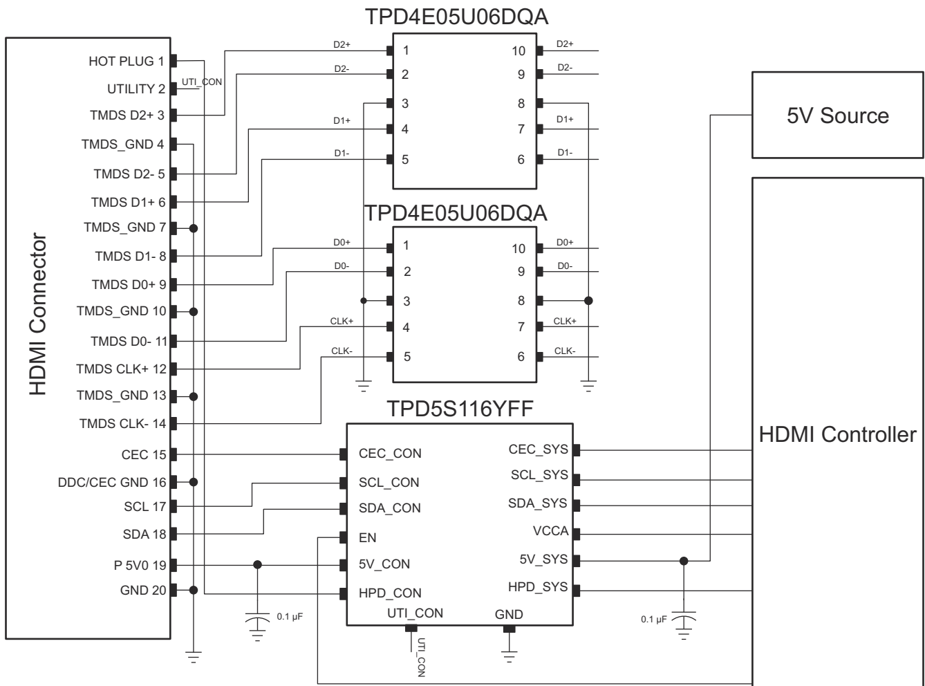
☒ 8-1. HDMI 2.0 Schematic
