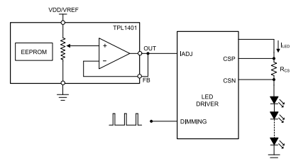
TPL1401 でプログラム可能な電流制限
