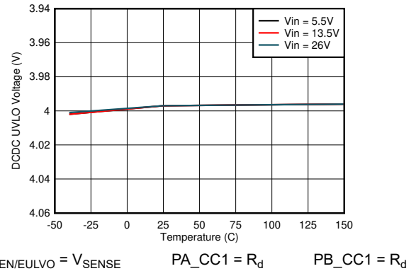
図 8-6. DCDC UVLO スレッシュホールド
