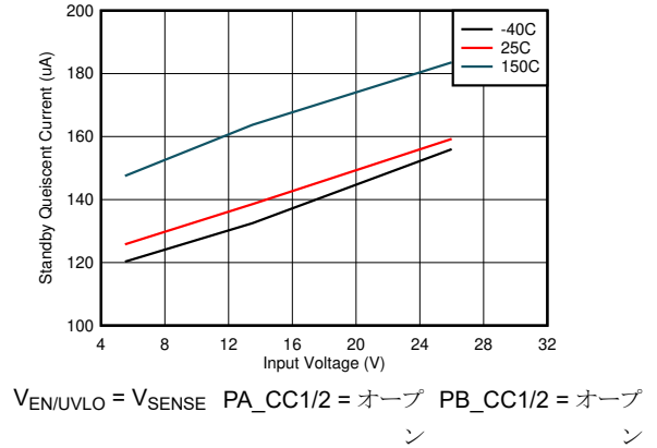
図 8-2. スタンバイ静止時電流
