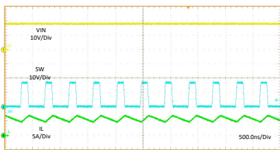
VIN = 18 V L = 0.68 \mu H I PA_BUS = 3 A I PB_BUS = 2.4 A
