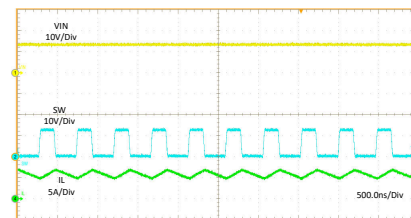
VIN = 13.5 V L = 0.68 \mu H I PA_BUS = 3 A I PB_BUS = 2.4 A
