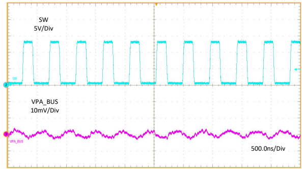
11-16. No Load Output Ripple
