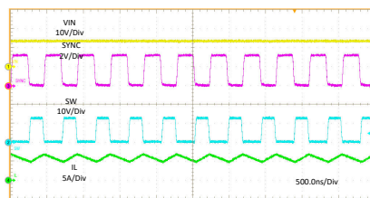
VIN = 13.5 V L = 0.68 \mu H I PA_BUS = 3 A I PB_BUS = 2.4 A
