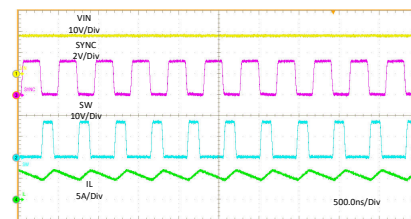
VIN = 18 V L = 0.68 \mu H I PA_BUS = 3 A I PB_BUS = 2.4 A
