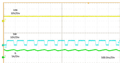
VIN = 8 V L = 0.68 \mu H I PA_BUS = 3 A I PB_BUS = 2.4 A
