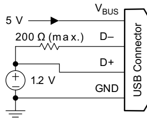
10-18. 1.2-V Mode
