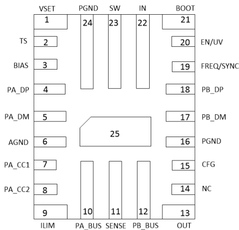
图 7-1. TPS25868 RPQ Package 25-Pin (QFN) Top View
