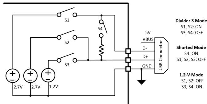
10-19. DCP Auto Mode
