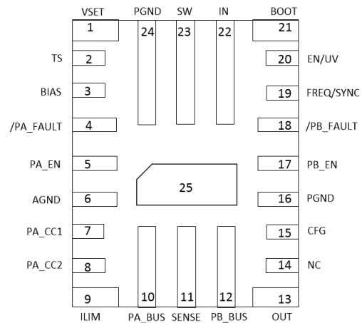
图 7-2. TPS25869 RPQ Package 25-Pin (QFN) Top View
