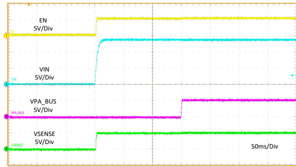
11-16. Startup Relate to VIN
