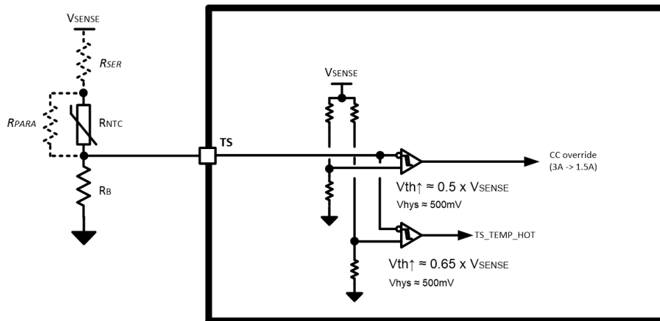
10-10. TS Input
