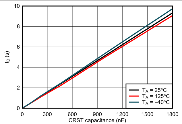
7-9. t_D vs Capacitance
