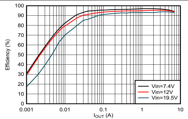
图 8-3. Efficiency, OOA Mode
