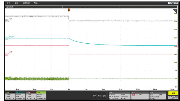
8-9. Shutdown Relative to EN Falling, Iout = 0A, OOA Mode
