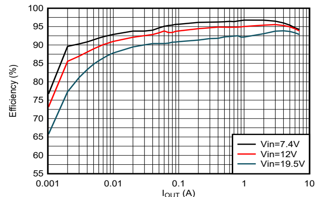
効率曲線、V OUT = 5.1V、PSM モード
