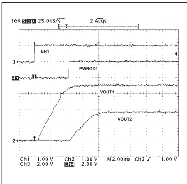
図 32. ENおよびPWRGDを使用したシーケンシャル・スタートアップ
