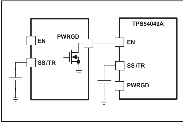
図 31. シーケンシャルなスタートアップ・シーケンスの回路図
