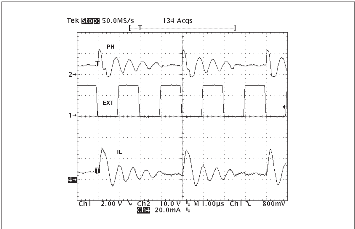
図 45. PSMでの同期プロット
