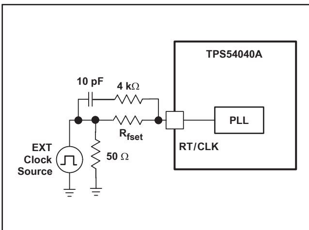
図 42. システム・クロックとの同期
