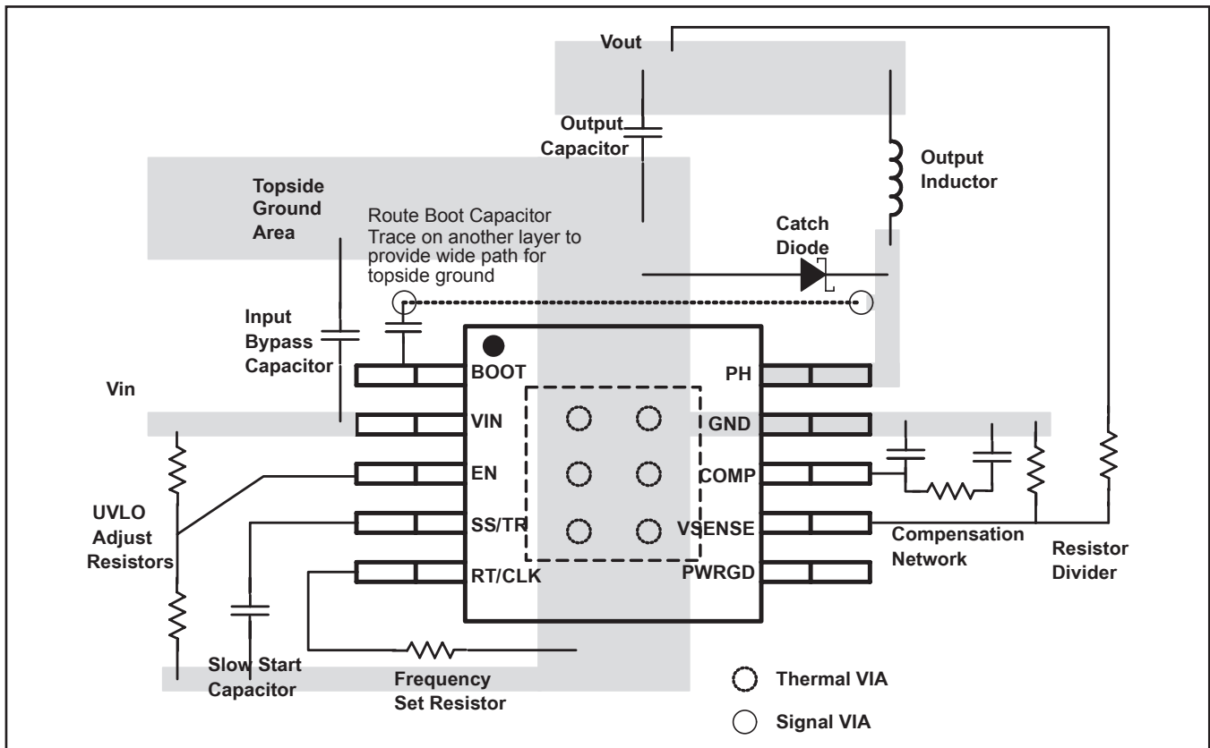
図 63. PCBレイアウト例
