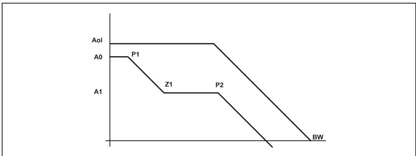
図 49. タイプ2Aおよびタイプ2B周波数補償の周波数応答
