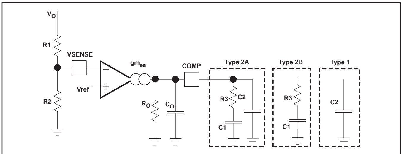
図 48. 周波数補償の種類
