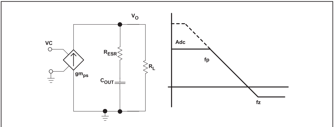
図 47. ピーク電流モード制御の単純な小信号モデルおよび周波数応答
