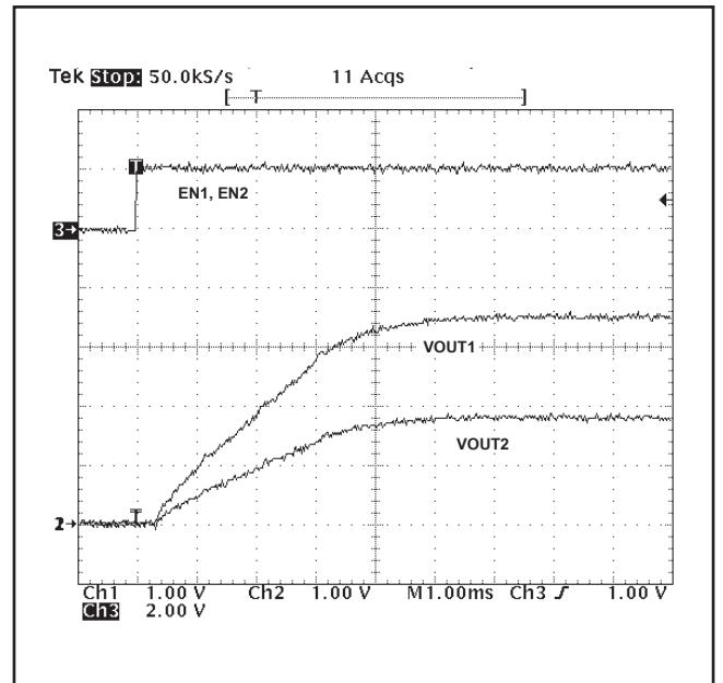
図 34. SS/TRピンの結合によるレシオメトリックなスタートアップ
