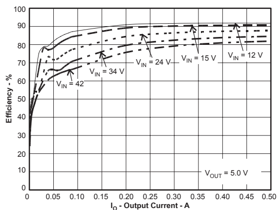
図 58. 効率 対 負荷電流
