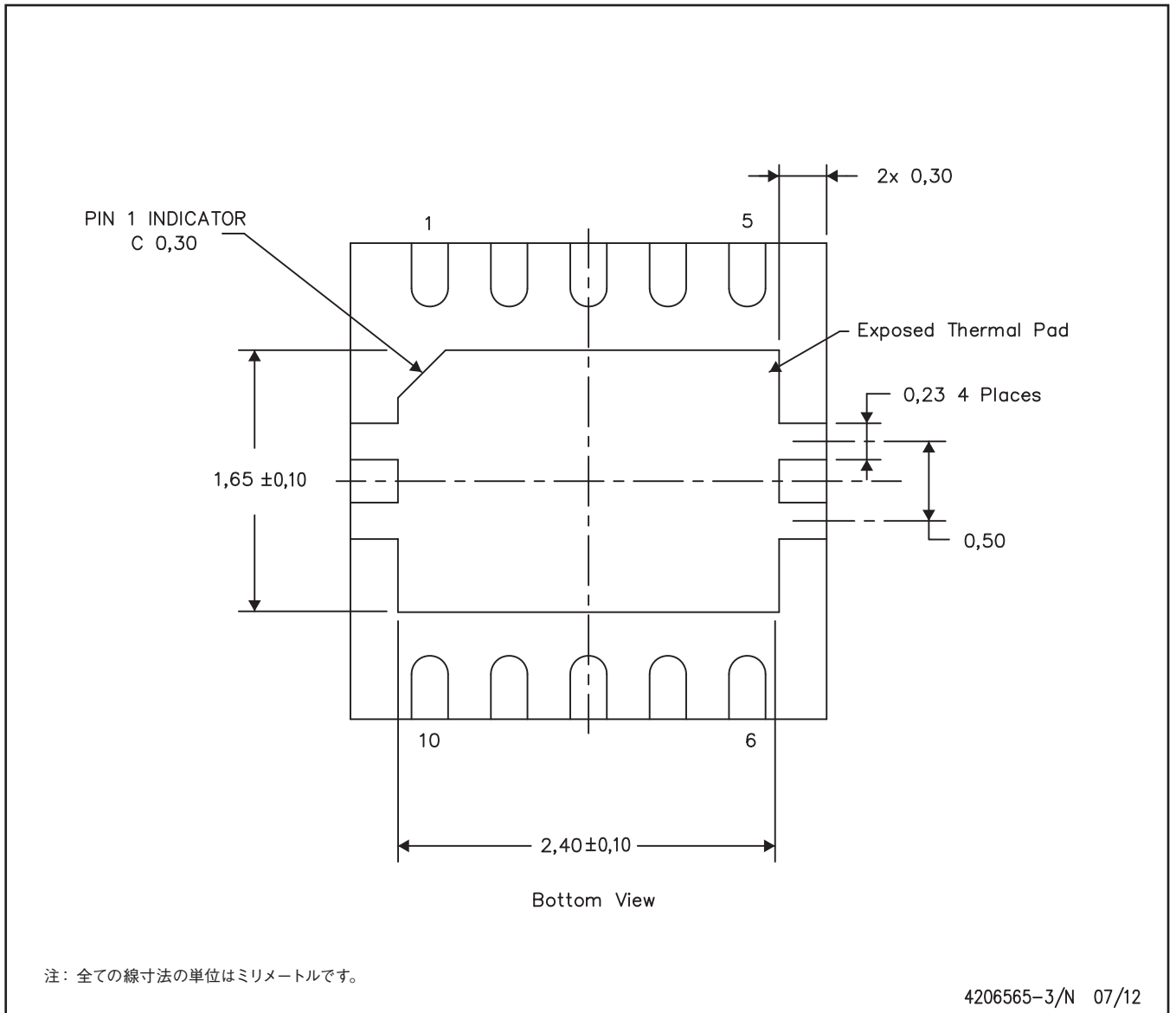
サーマルパッド寸法図
