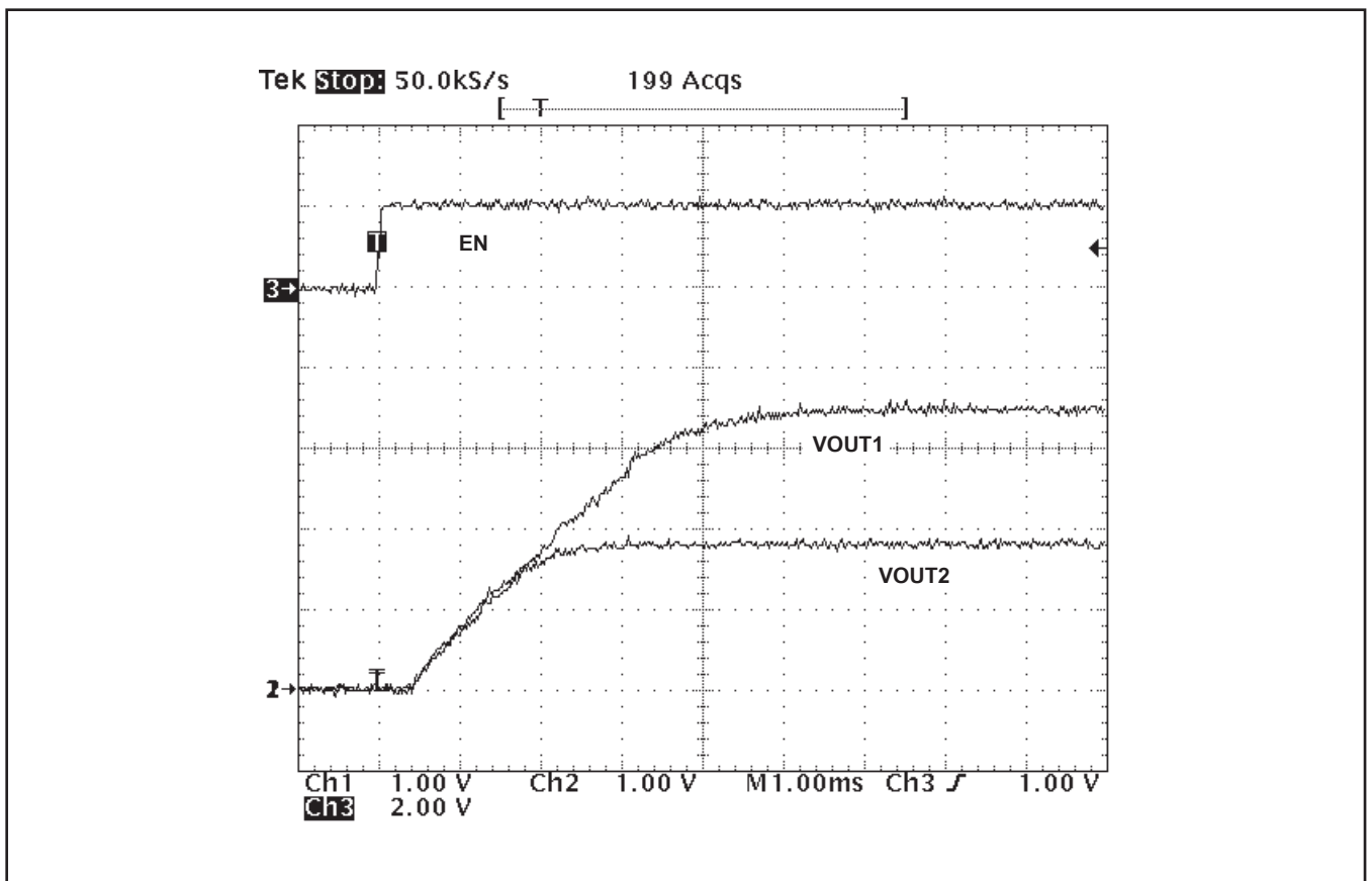
図 38. トラッキング抵抗による同時スタートアップ
