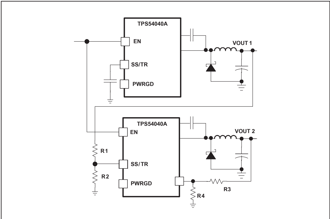
図 35. レシオメトリックな同時スタートアップ・シーケンスの回路図
