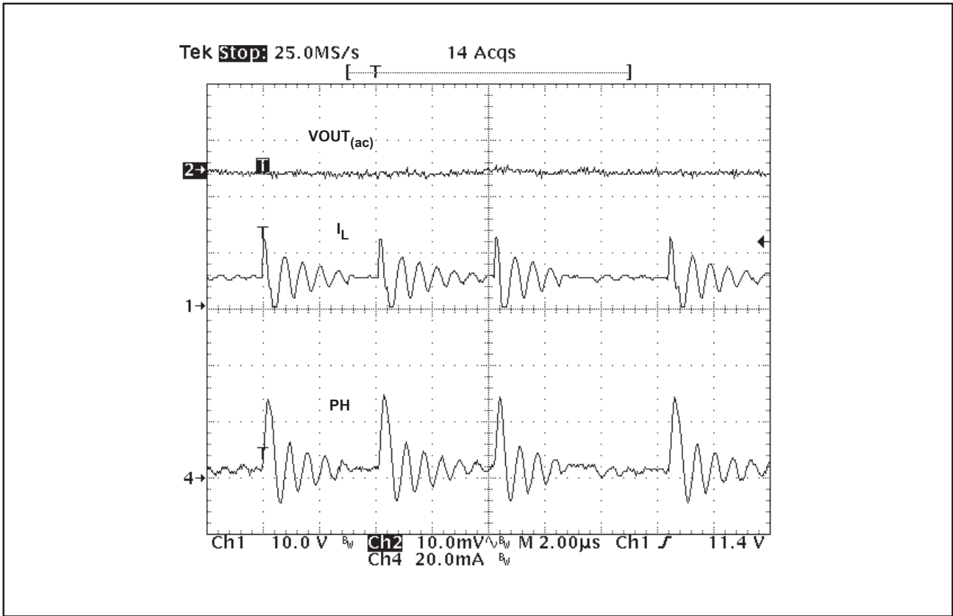
図 25. パルス・スキップ・モードの動作
