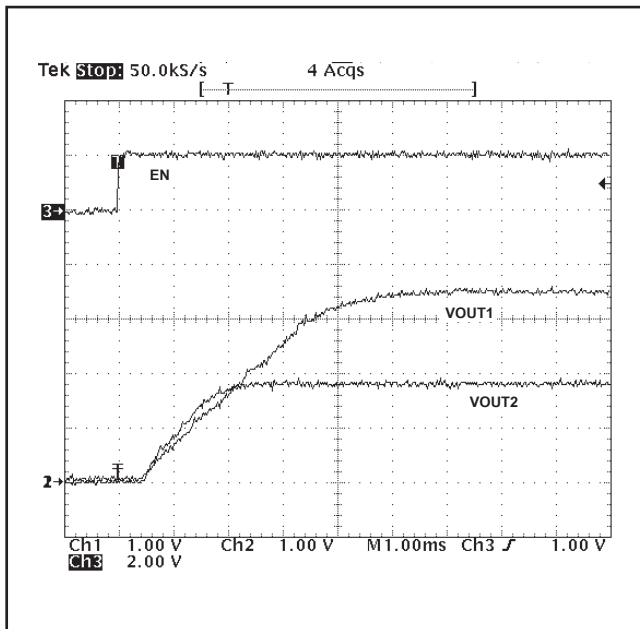
図 36. トラッキング抵抗によるレシオメトリックなスタートアップ
