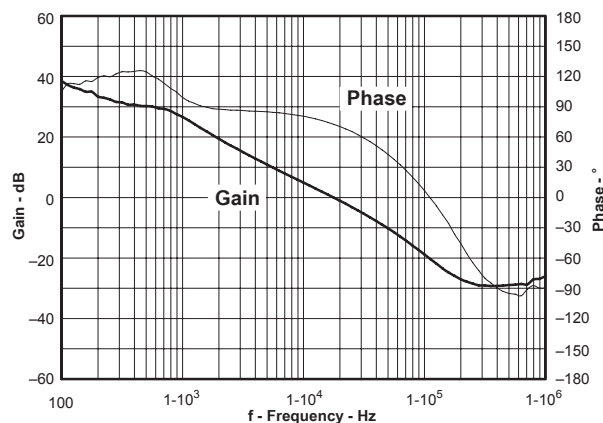
図 60. ループ全体の周波数応答
