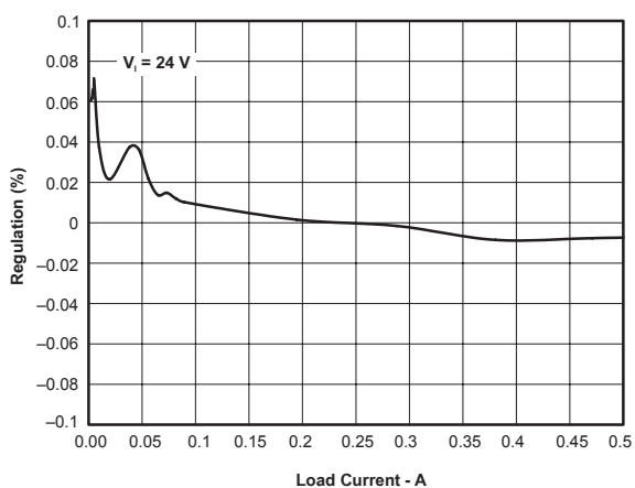
図 61. レギュレーション 対 負荷電流
