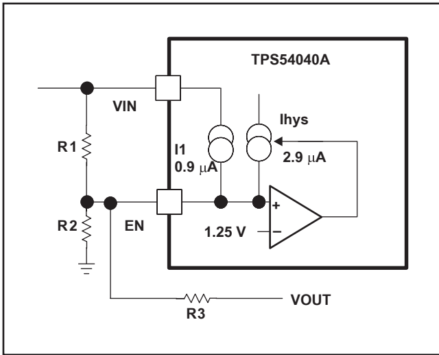
図 29. 追加ヒステリシスの提供
