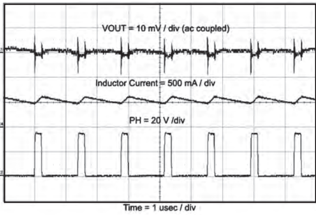
図 53. 出力リップルCCM
