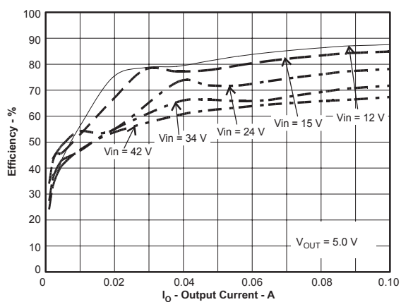
図 59. 軽負荷効率
