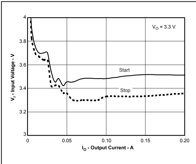
図 26. 3.3Vアプリケーションの開始/停止電圧
