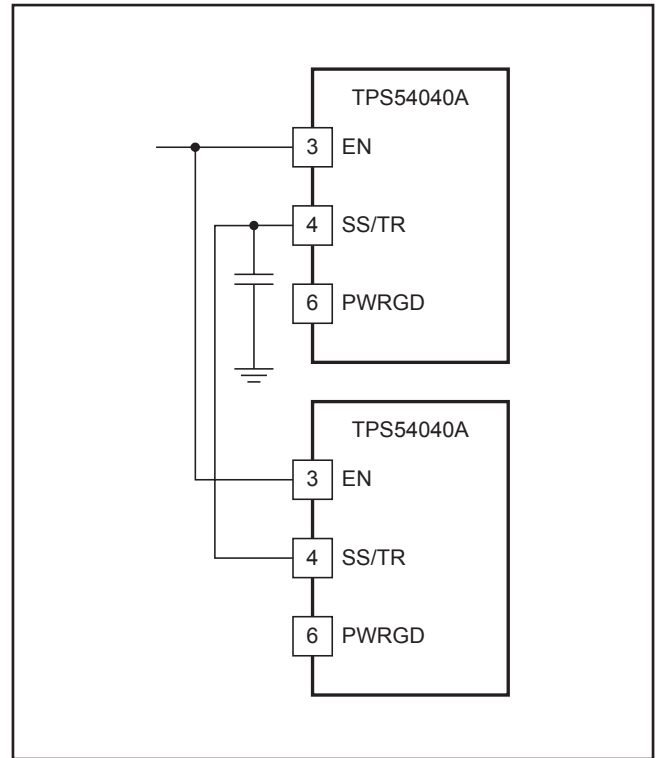
図 33. レシオメトリックなスタートアップ・シーケンスの回路図
