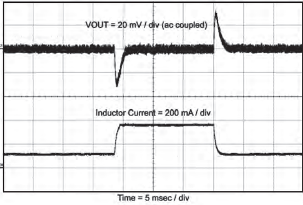
図 51. 負荷過渡応答
