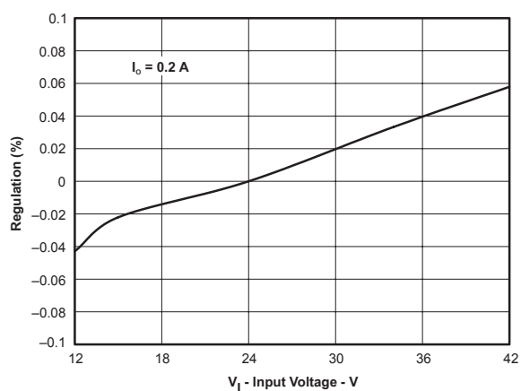
図 62. レギュレーション 対 入力電圧
