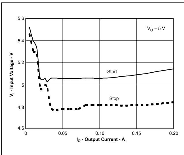
図 27. 5.0Vアプリケーションの開始/停止電圧
