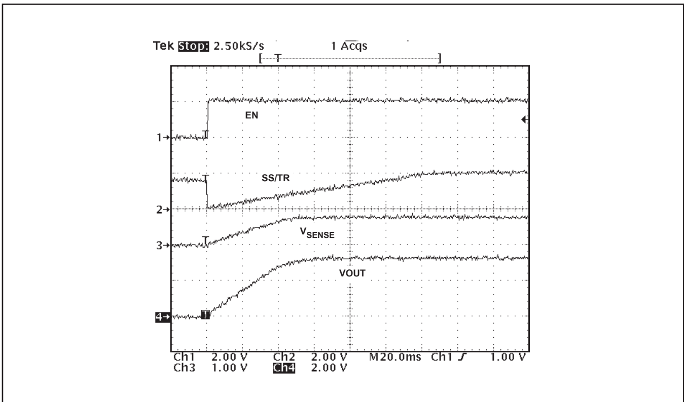
図 30. 起動時のSS/TRピンの動作
