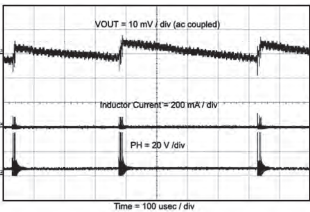
図 55. 出力リップルPSM
