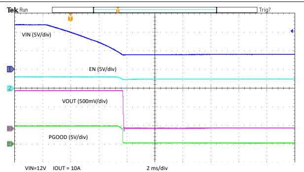
7-15. VIN Shutdown
