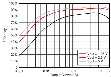
TPS562202S の効率
