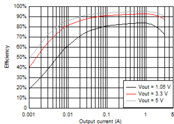
TPS563202S の効率
