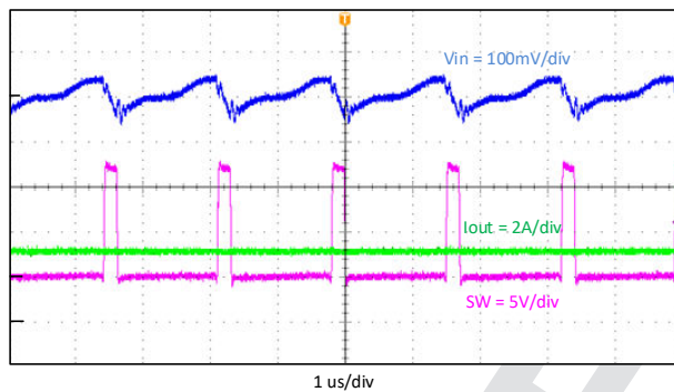
☒ 9-4. Input Voltage Ripple
