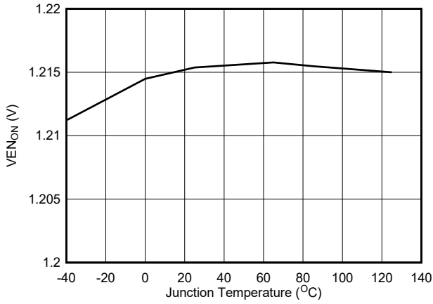
图 5-3. Enable On Threshold Voltage
