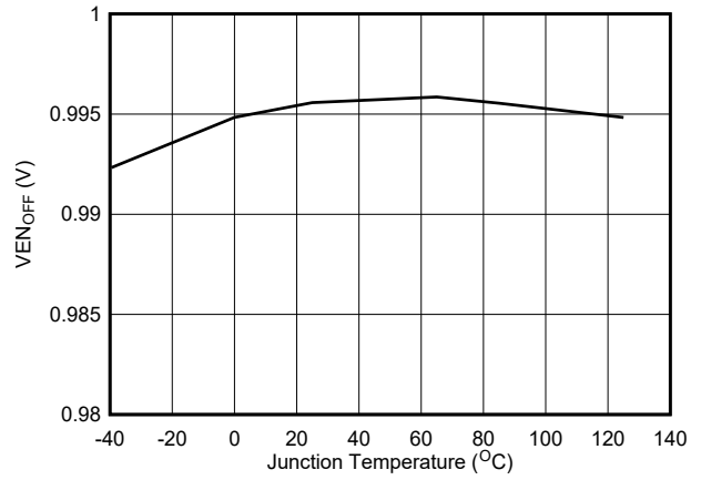
图 5-4. Enable Off Threshold Voltage
