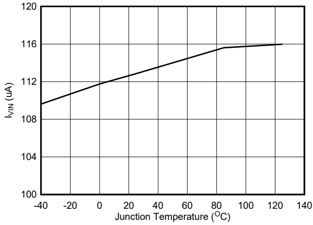
图 5-1. TPS563203 Quiescent Current
