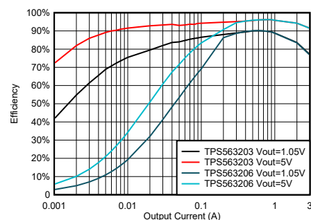
TPS563203 と TPS563206 の効率
