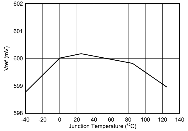
图 5-2. V_{ref} Voltage
