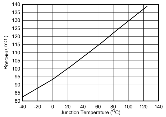
图 5-6. High-Side R_{dson}
