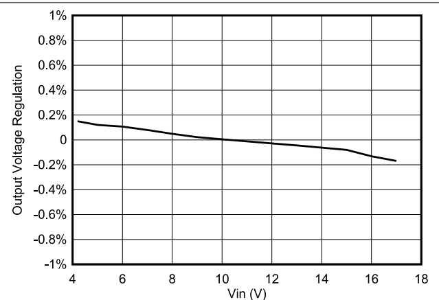
7-7. TPS563206 Line Regulation vs Vin at 1-A Loading
