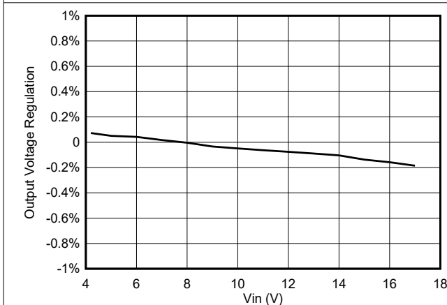
7-6. TPS563203 Line Regulation vs Vin at 1-A Loading
