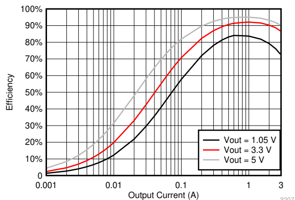
TPS563207S の効率
