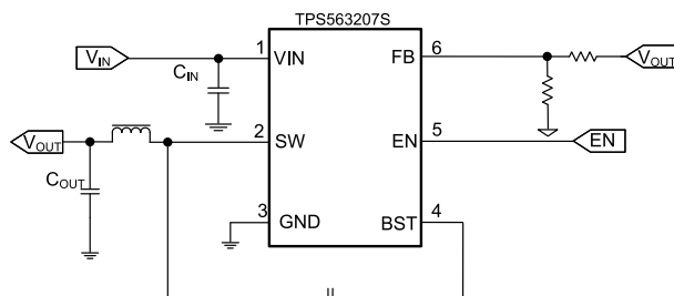
概略回路図
