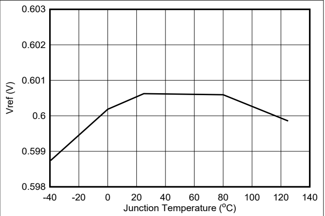
6-8. VREF Voltage
