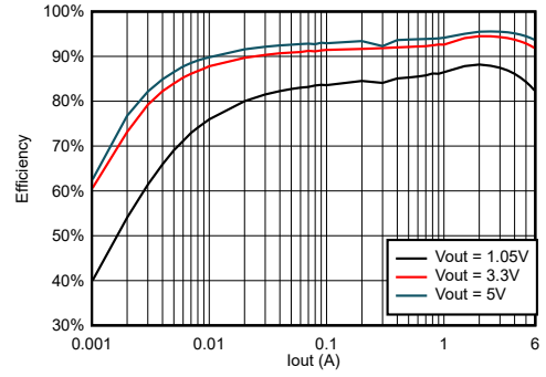
TPS566242 の効率 ( V_{IN} = 12V )
