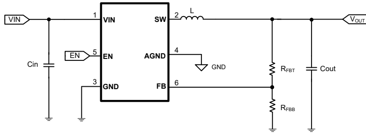
概略回路図
