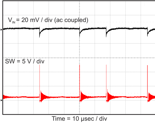
8-8. Input Voltage Ripple, I_{OUT} = 10\text{ mA}
