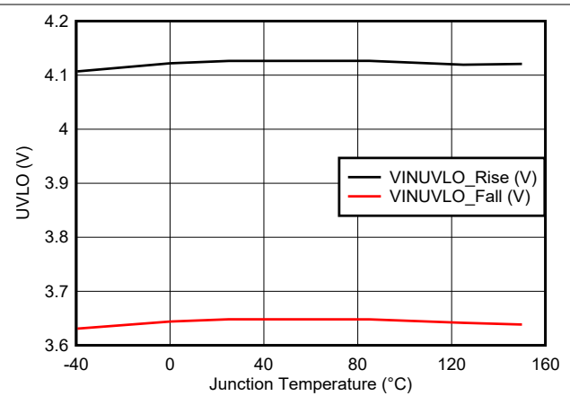
5-6. VIN UVLO vs Temperature
