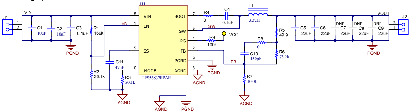
図 7-1. TPS56837 5V, 8A Reference Design
