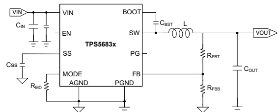
概略回路図
