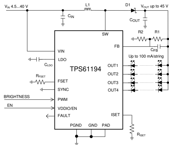
概略回路図
