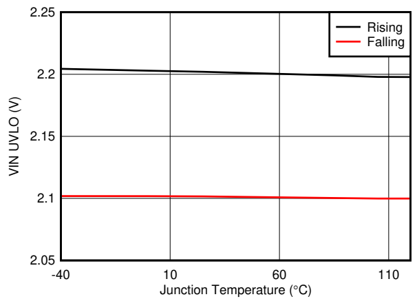
7-16. VIN UVLO vs Temperature
