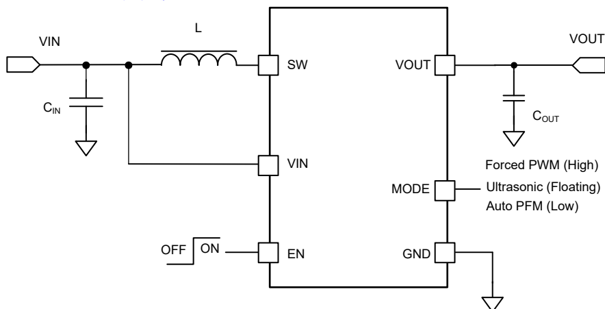
代表的な回路図
