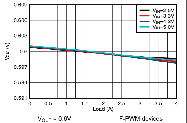
図 8-6. Load Regulation
