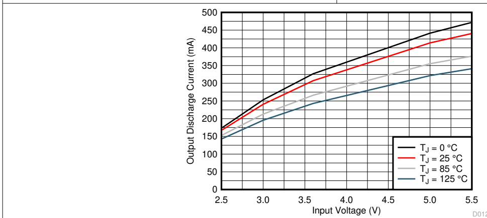
图 6-5. Output Discharge Current
