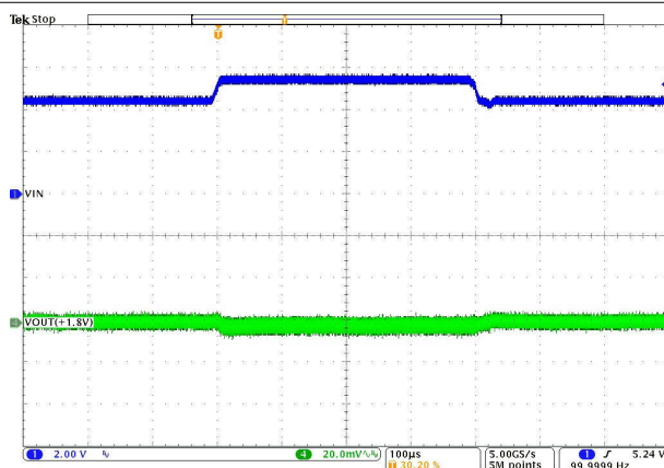
図 8-35. Load Transient
