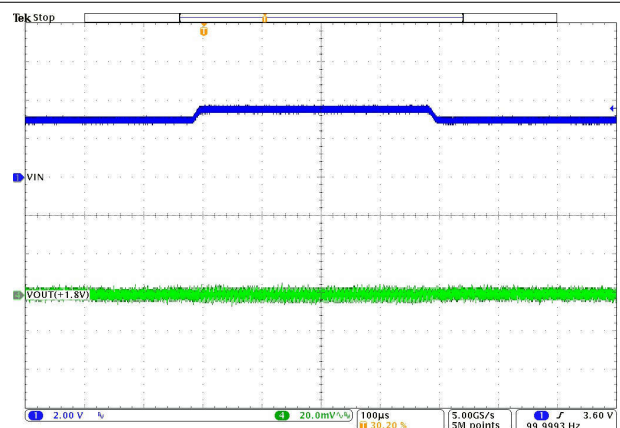
図 8-36. Line Transient
