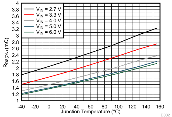
図 6-2. R_{DS(ON)} of Low Side Switch
