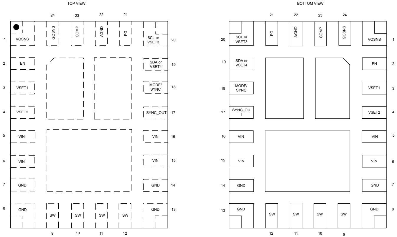
図 5-1. RZV Package 24 Pin VQFN
