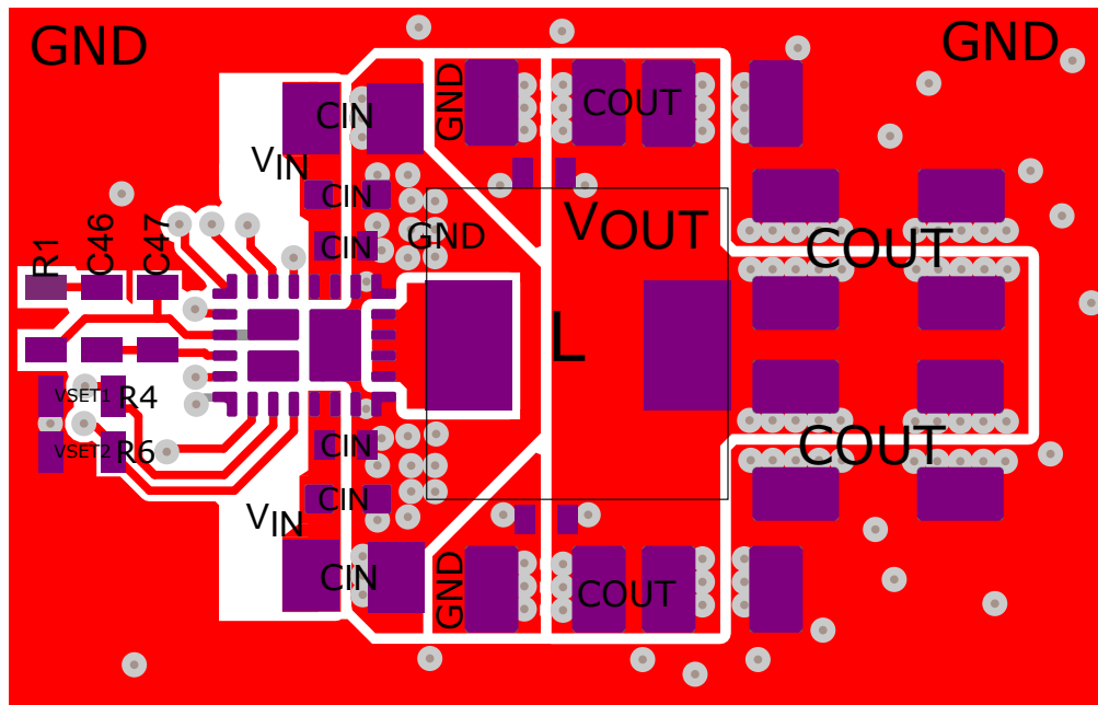
☒ 9-40. TPS6287B25 EVM Top Layer
