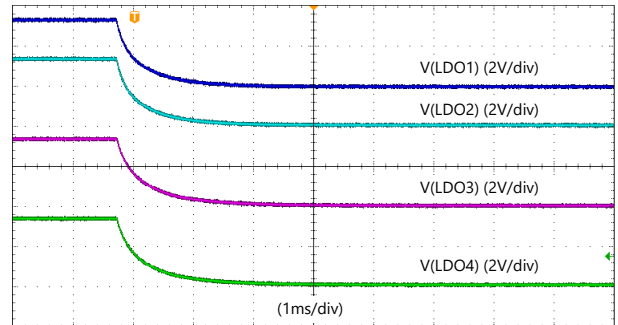
7-9. LDOs Discharge
