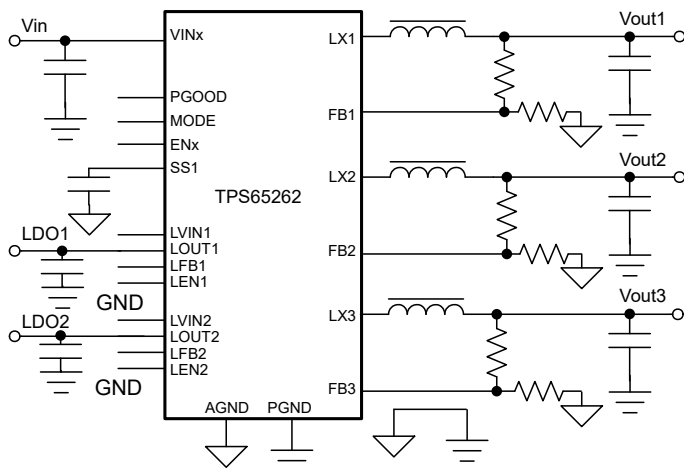
アプリケーション回路図
