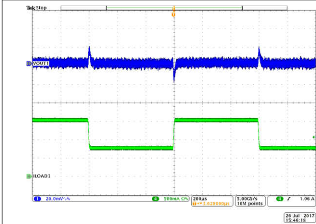
8-9. BUCK1 Load Transient
