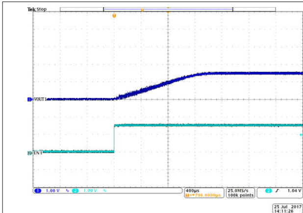
8-3. BUCK1 Soft-Start
