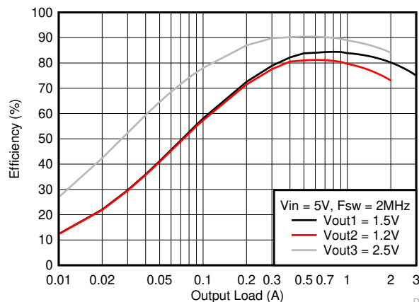
効率と出力負荷との関係
