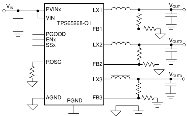
アプリケーション回路図
